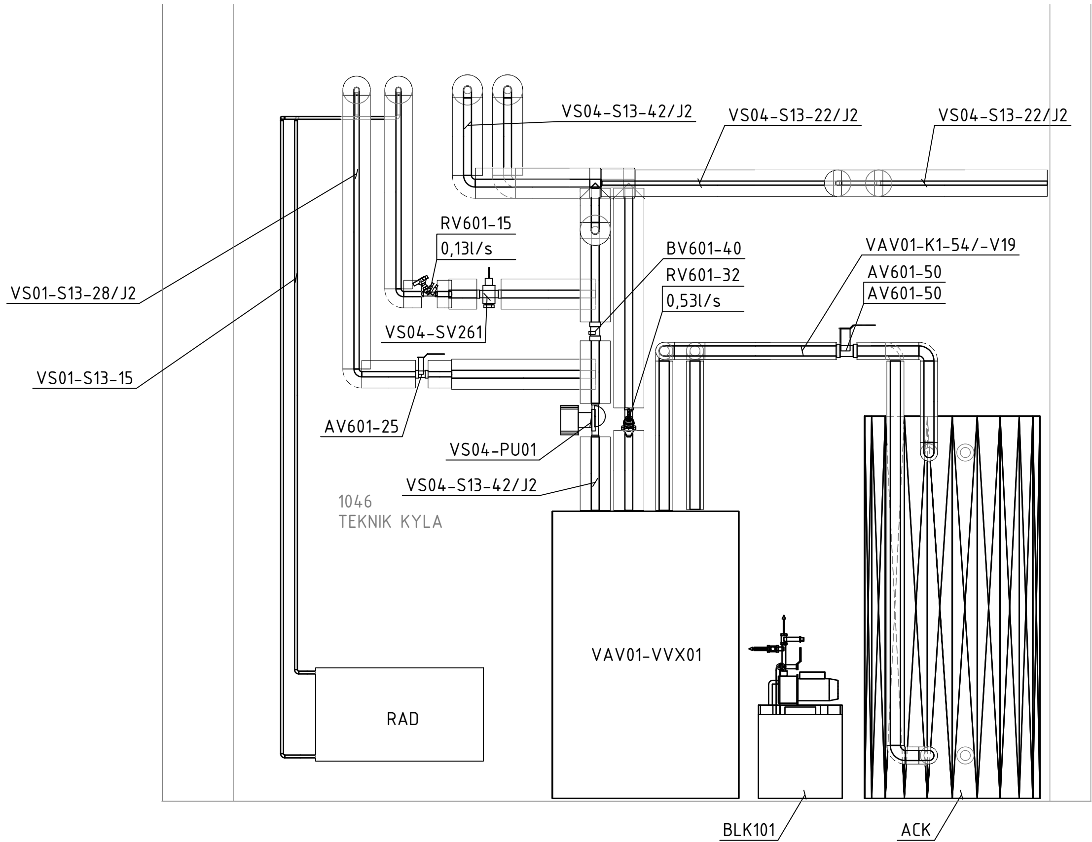
SEKTION 10 KYLCENTRAL SKALA 1:20
